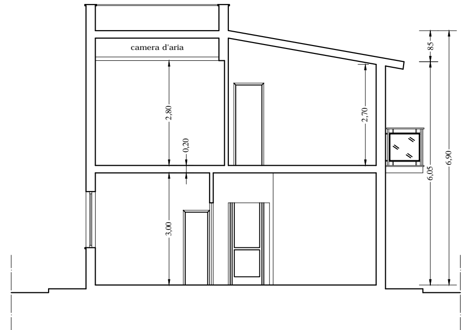
SEZIONE "X-X" Scala 1:100
