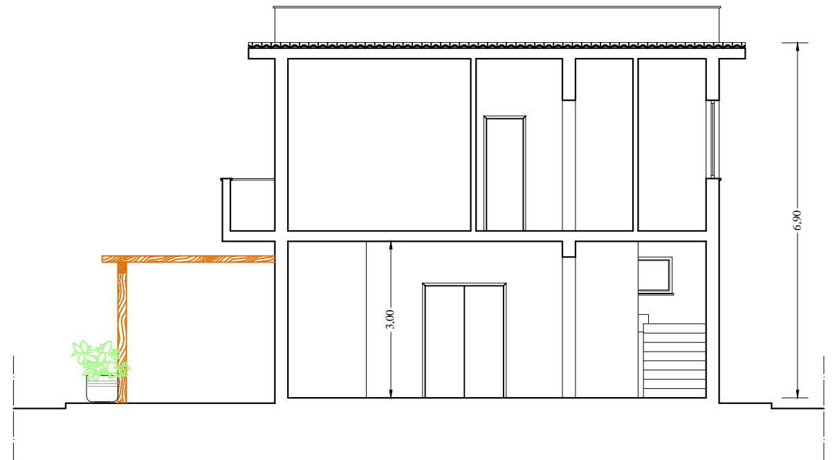
SEZIONE "Y-Y" Scala 1:100
