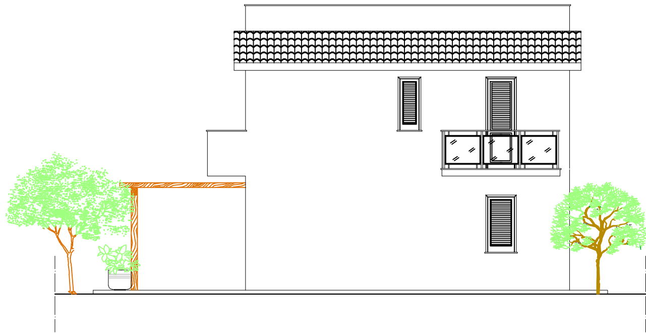
PROSPETTO "D" Scala 1:100
